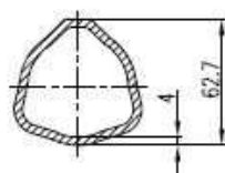
Tubo exterior
