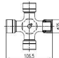
Cruceta
