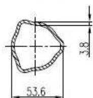
Tubo exterior
