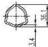
Tubo exterior
